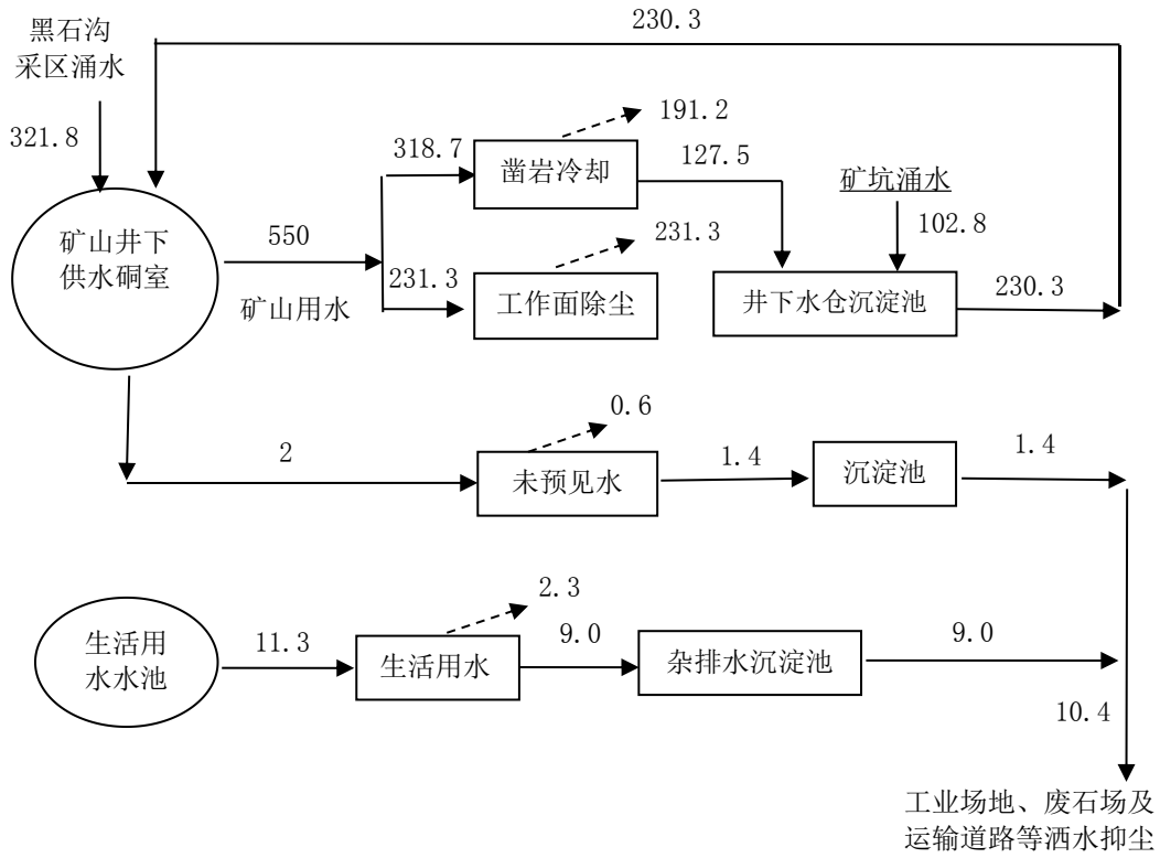
图 3.3.2-1 水闸东沟采区用排水水量平衡图 单位: \text{m}^3/\text{d}
