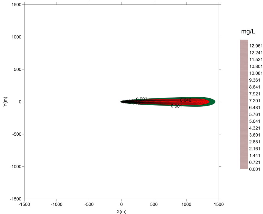
图 9.8.2-5 尾矿库渗漏铅在第四系含水层运移 1000d
