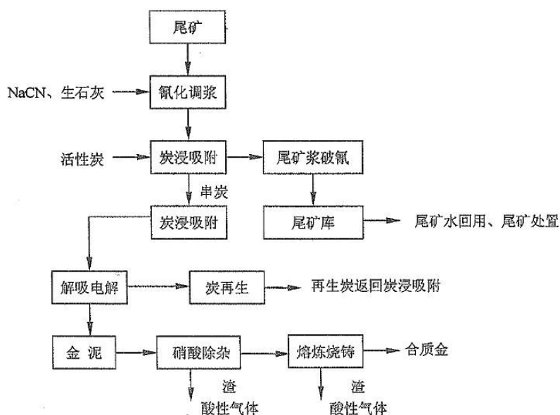
图 2.4.2-2 尾矿提金工艺流程图
