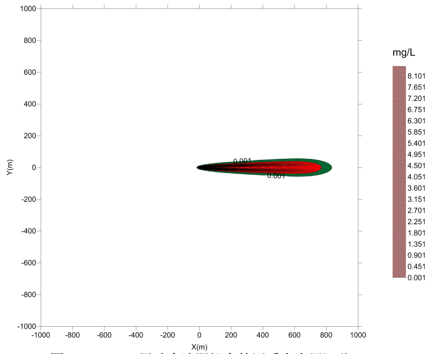
图 9.8.2-4 尾矿库渗漏铅在第四系含水层运移 200d
