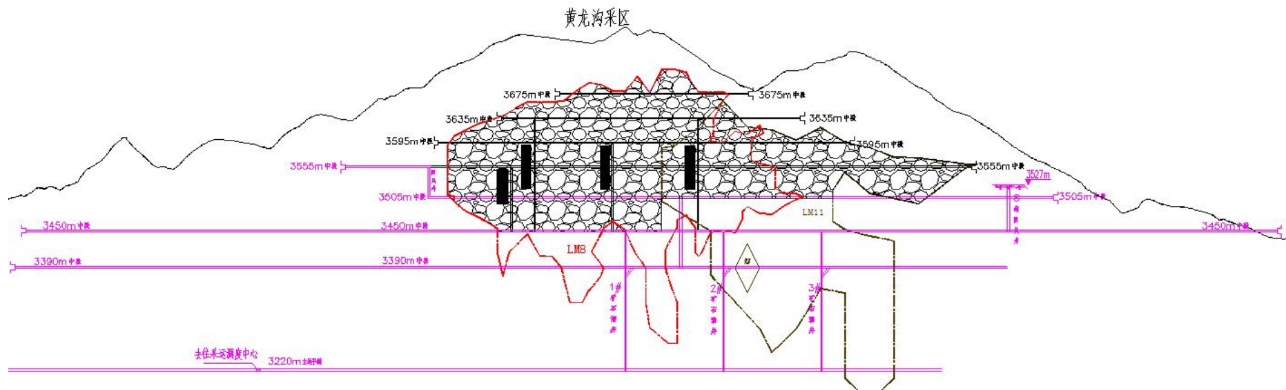
图 2.4.1-3 黄龙沟采区开拓系统垂直纵投影现状图
