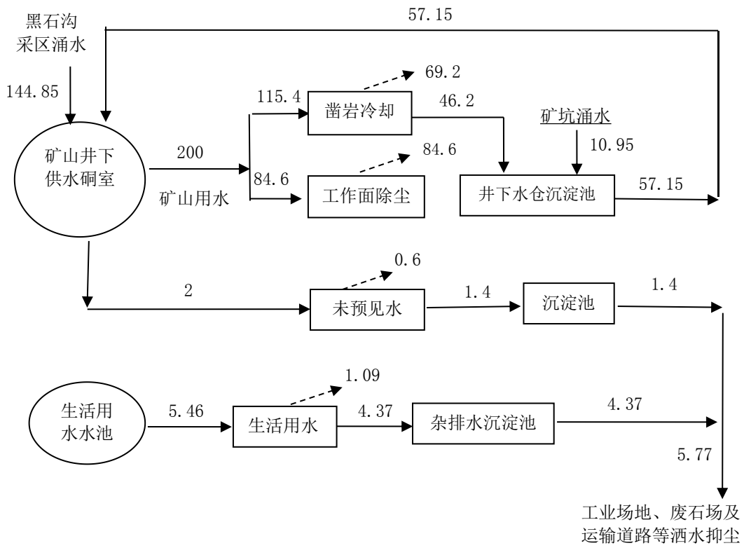
图 3.3.2-2 黄龙沟采区用排水水量平衡图 单位: \text{m}^3/\text{d}
