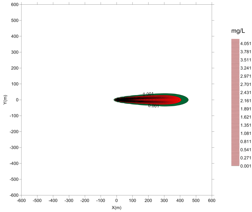
图 9.8.2-3 尾矿库渗漏铅在第四系含水层运移 100d
