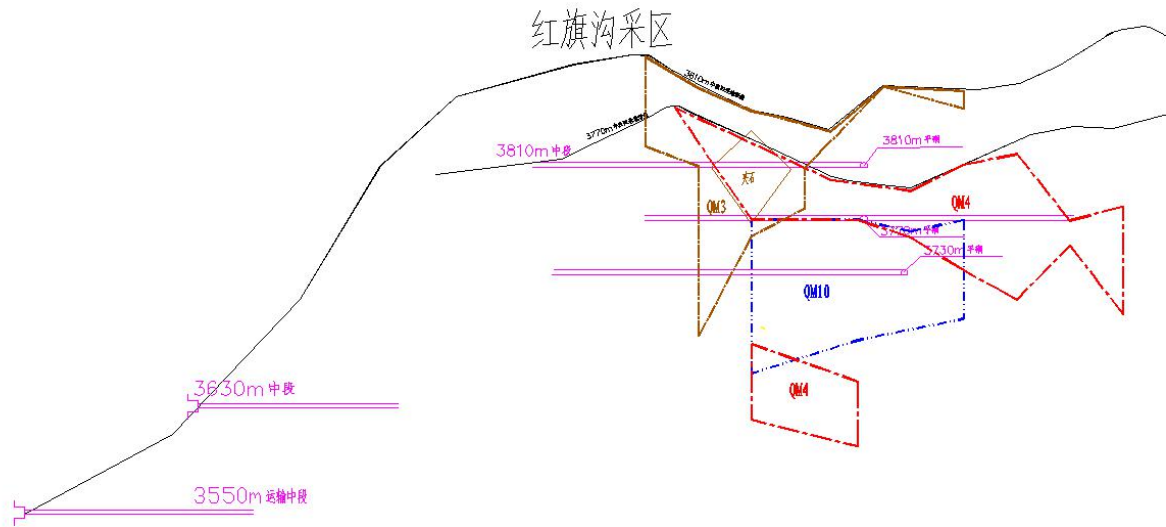
图 2.4.1-5 红旗沟采区开拓系统垂直纵投影现状图
