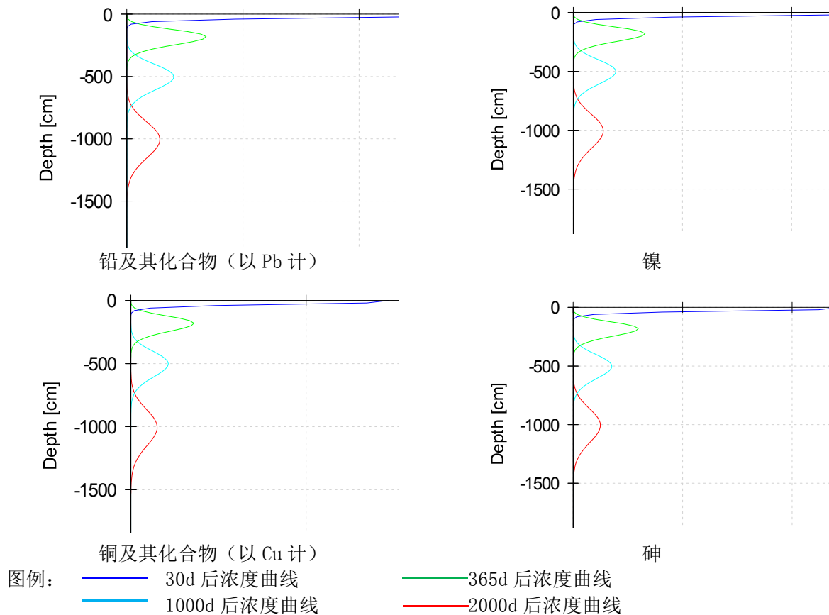
图 8.3.1-1 渗漏事故后土壤重金属浓度预测曲线图
