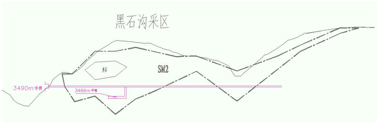
图 2.4.1-4 黑石沟采区开拓系统垂直纵投影现状图
