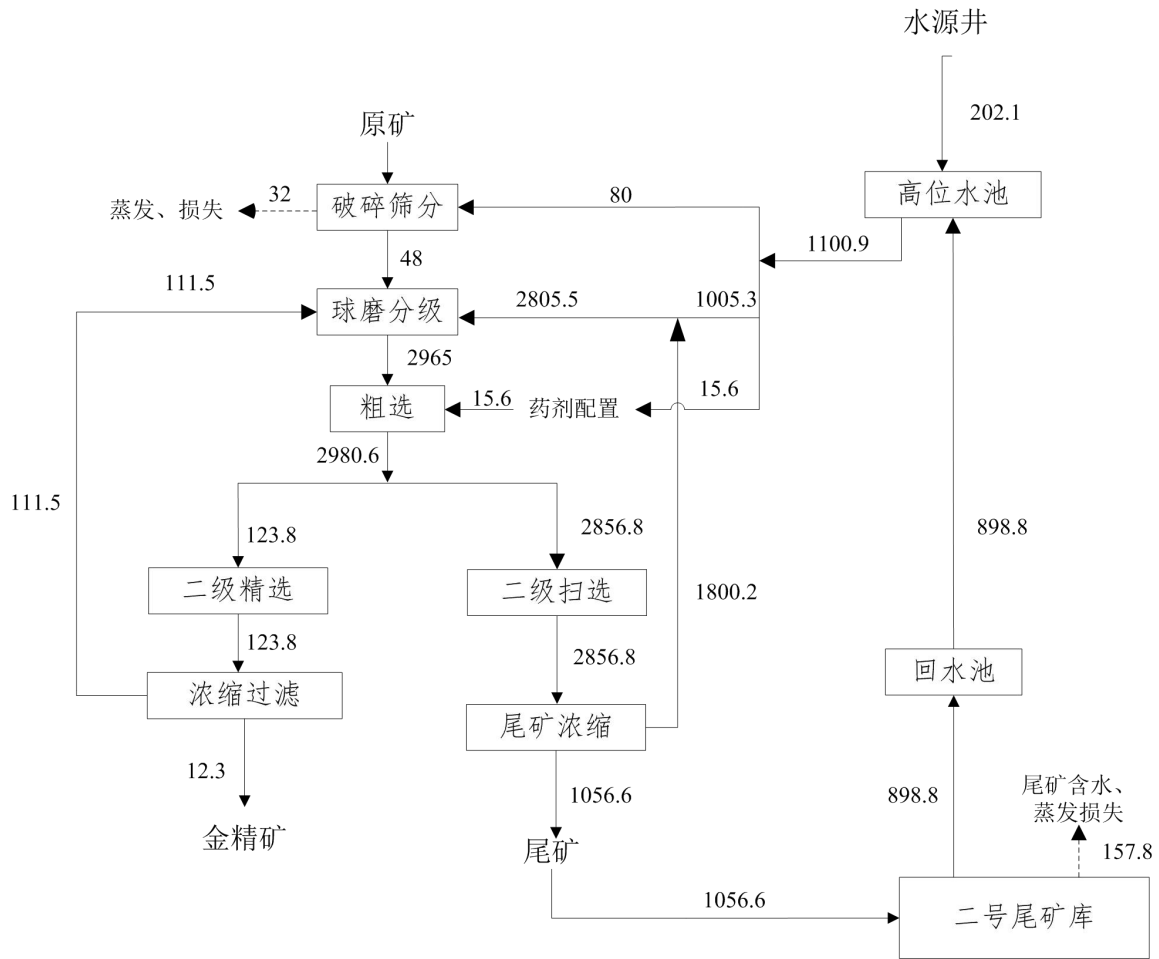
图 3.3.2-5 一选厂改扩建后用排水水平衡图 单位: m 3 /d
