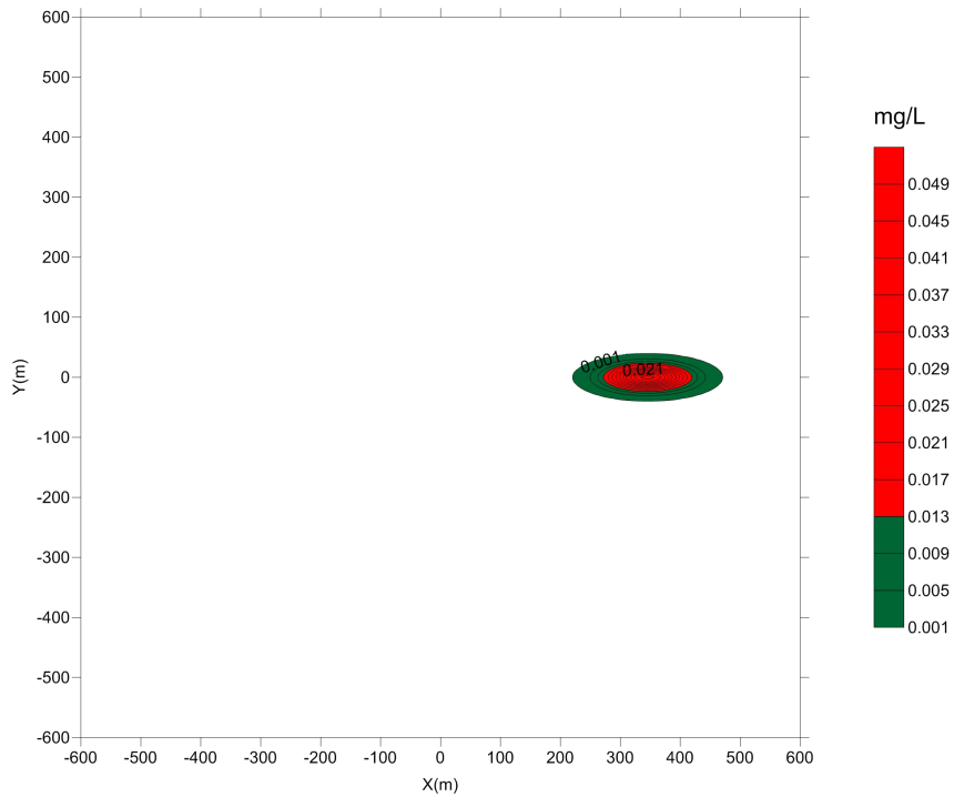
图 9.8.2-1 浓缩池渗漏铅在第四系潜水含水层运移 100d
