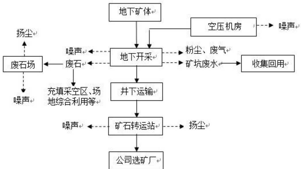
图 3.2.1-1 矿山采矿工艺流程及产污环节分布图
