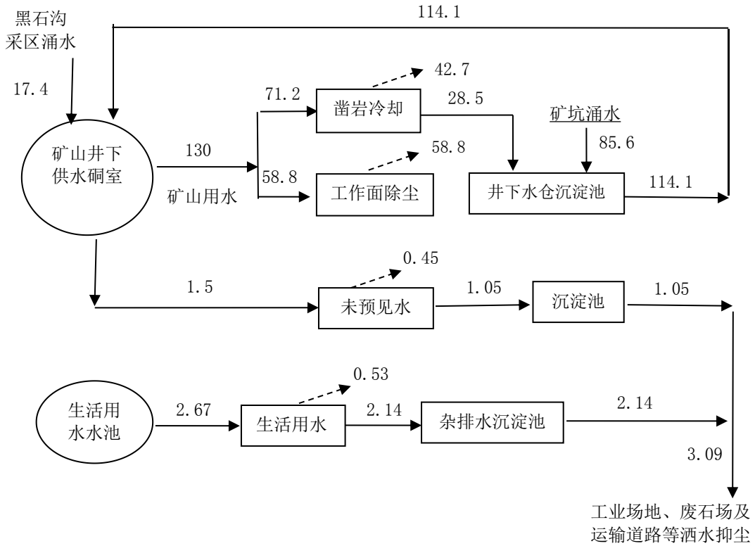
图 3.3.2-4 红旗沟采区用排水水量平衡图 单位: m 3 /d
