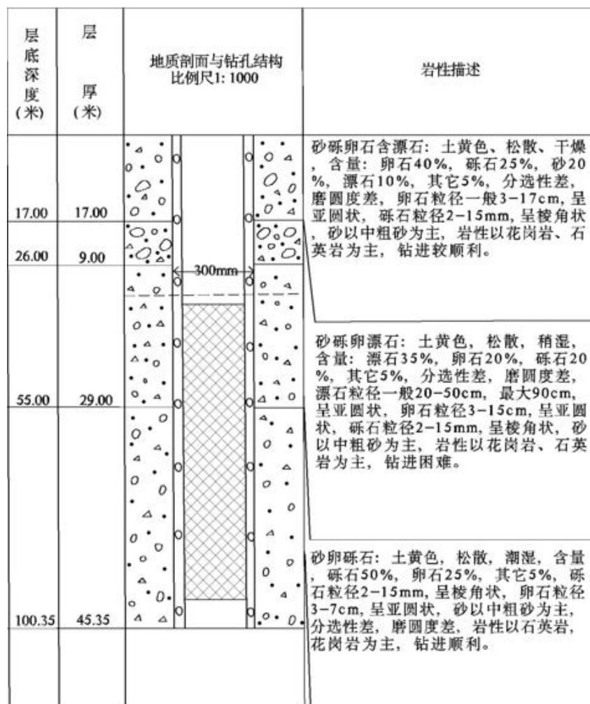
图 9.10.2-2 尾矿库下游监测井结构图
