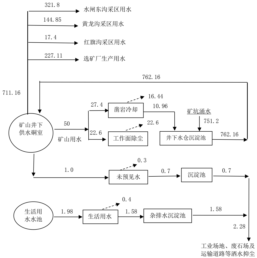
图 3.3.2-3 黑石沟采区用排水水量平衡图 单位: m^3/d
