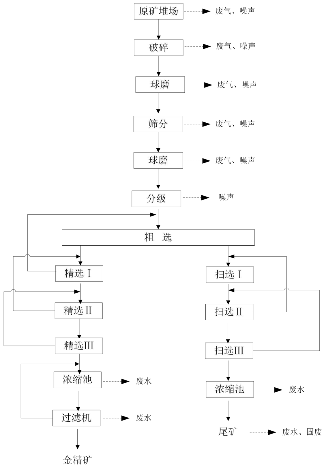
图 3.2.1-3 二选厂工艺流程及产物环节图
