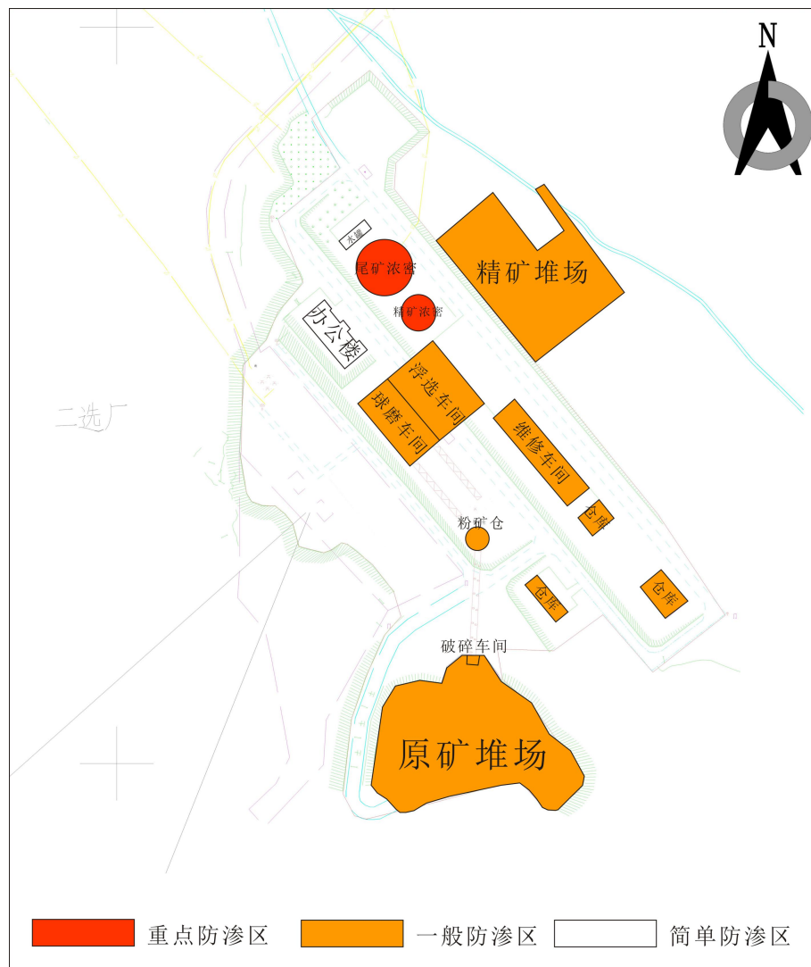
图 9.10.2-2 二选厂防渗分区图
