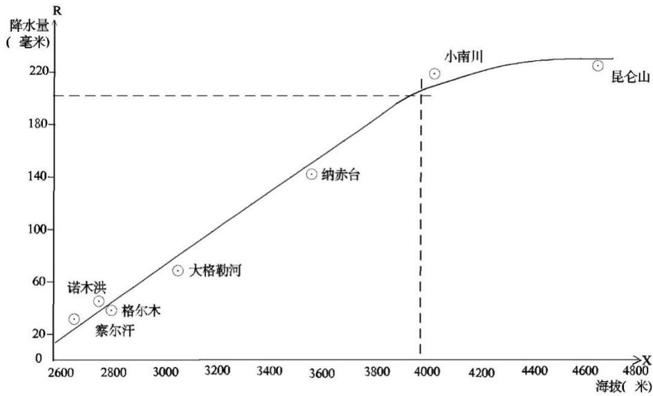
图 9.4.2-1 降水量随海拔高度变化图
