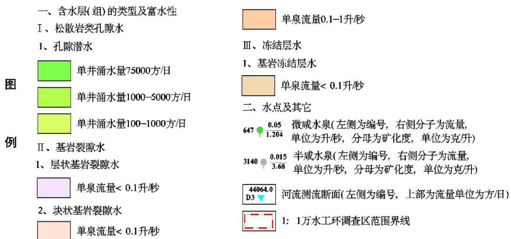
图 9.5.1-1 区域水文地质图
