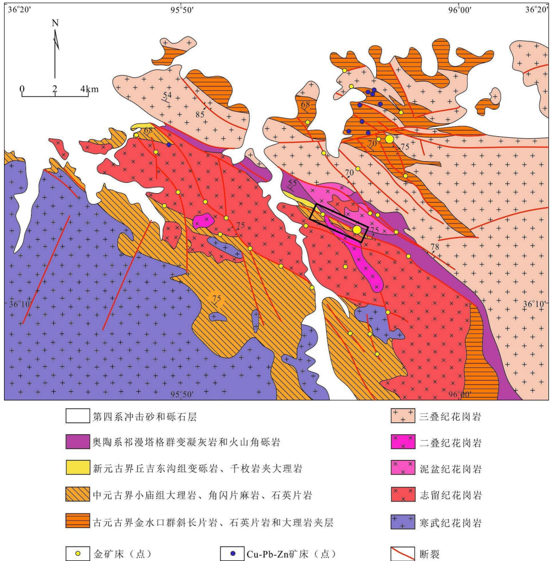
图 9.4.4-1 东昆仑五龙沟矿集区地质简图
