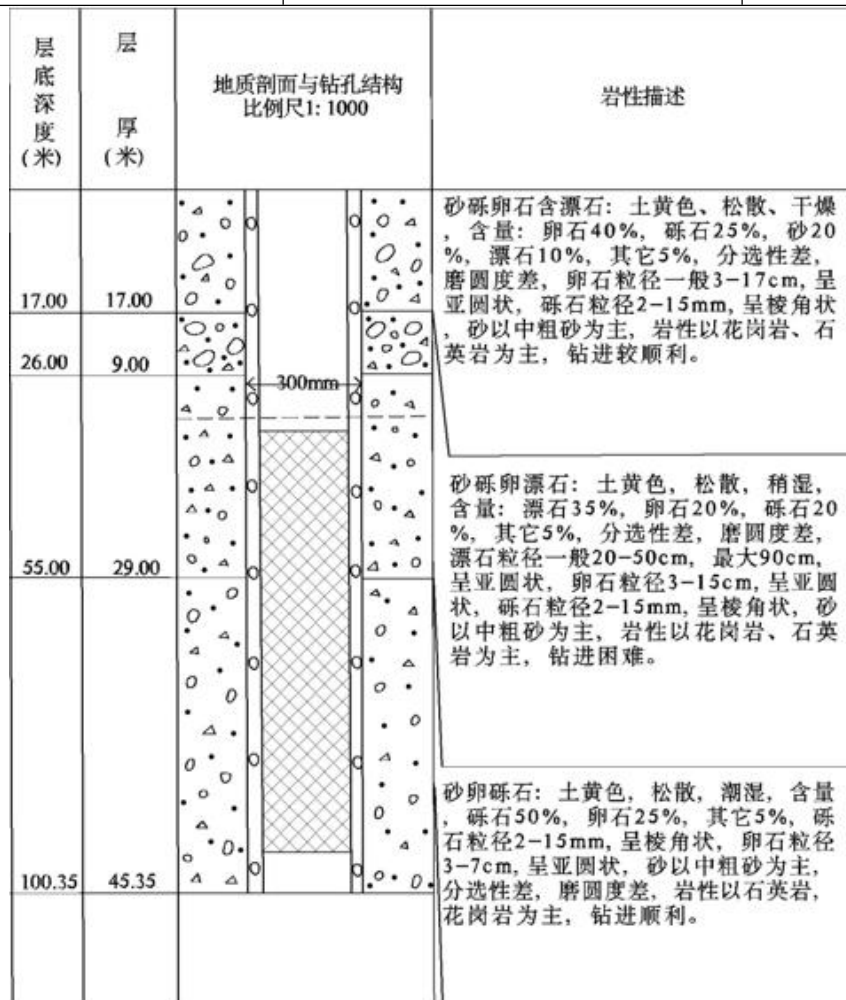
图 9.10.2-4 尾矿库周边监测井结构图
