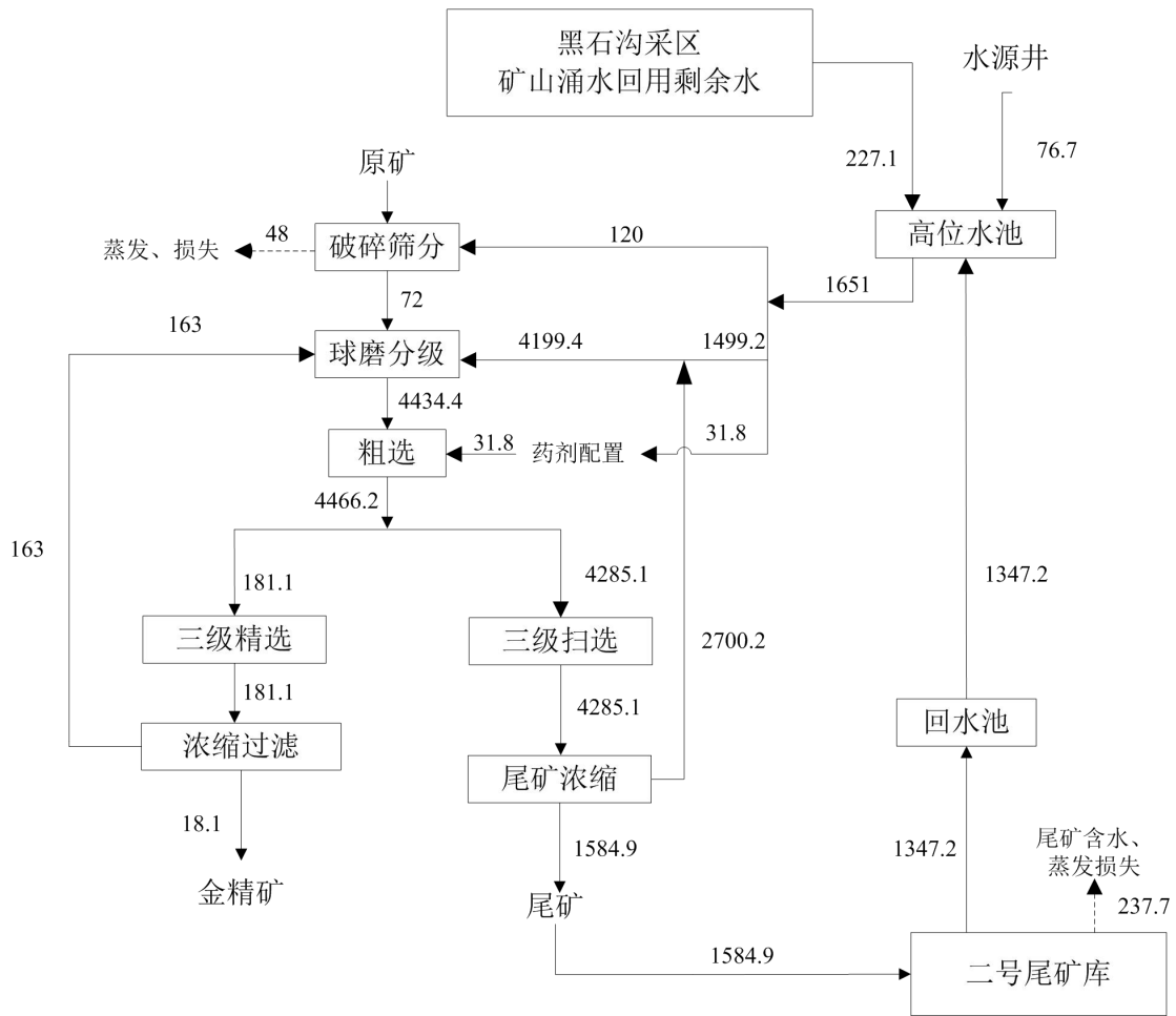
图 3.3.2-6 二选厂改扩建后用排水水平衡图 单位: \text{m}^3/\text{d}
