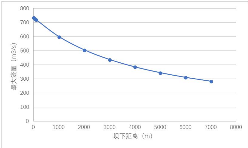
图6.8.5-1 溃坝最大流量沿程演进曲线图
