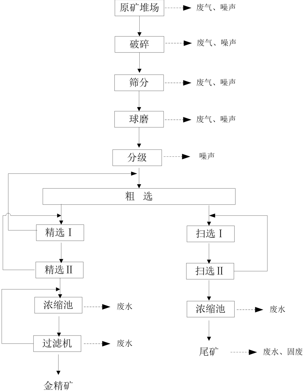
图 3.2.1-2 一选厂工艺流程及产物环节图
