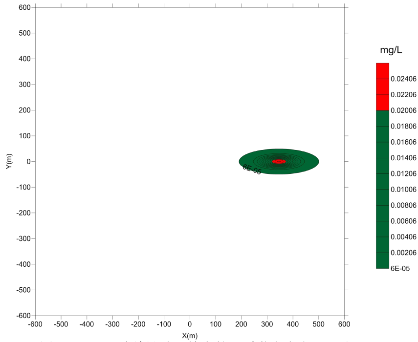
图 9.8.2-3 浓缩池渗漏镍在第四系潜水含水层运移 100d
