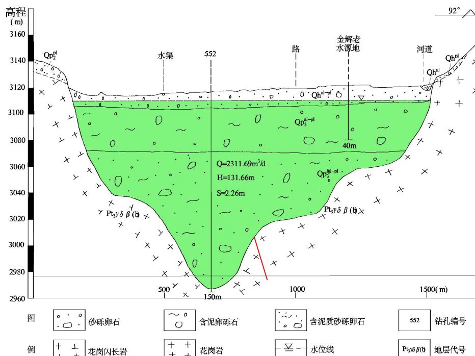
图 9.5.1-2 五龙沟沟口水文地质剖面图 (该剖面位于二选厂及尾矿库下游)
