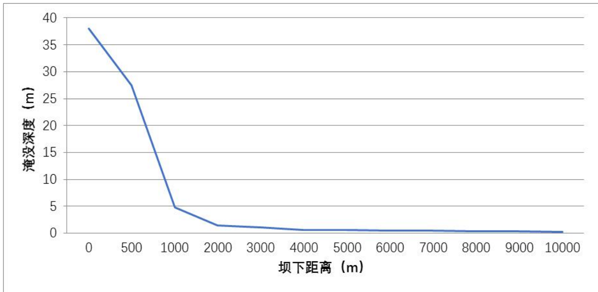
图6.8.5-2 溃坝后尾砂淹没深度沿程演进曲线图
