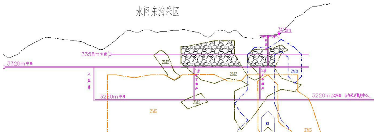
图 2.4.1-1 水闸东沟采区开拓系统垂直纵投影现状图
