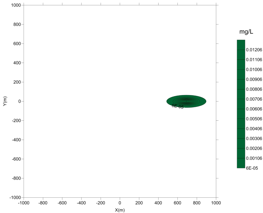
图 9.8.2-4 浓缩池渗漏镍在第四系潜水含水层运移 200d
