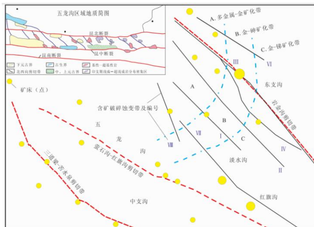
图 9.4.5-1 红旗沟—深水潭金矿区域地质构造图
