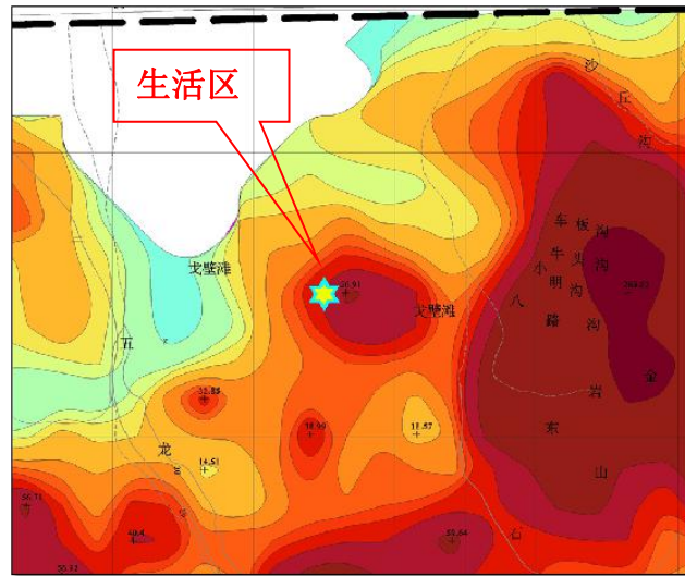
图 4.3.5-1 五龙沟地区 1:5 万 AS 元素地球化学图
