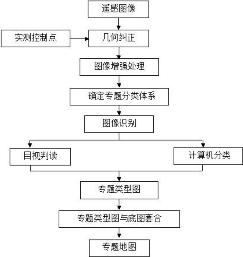
图 4.2.1-1 遥感影像解译处理流程图
