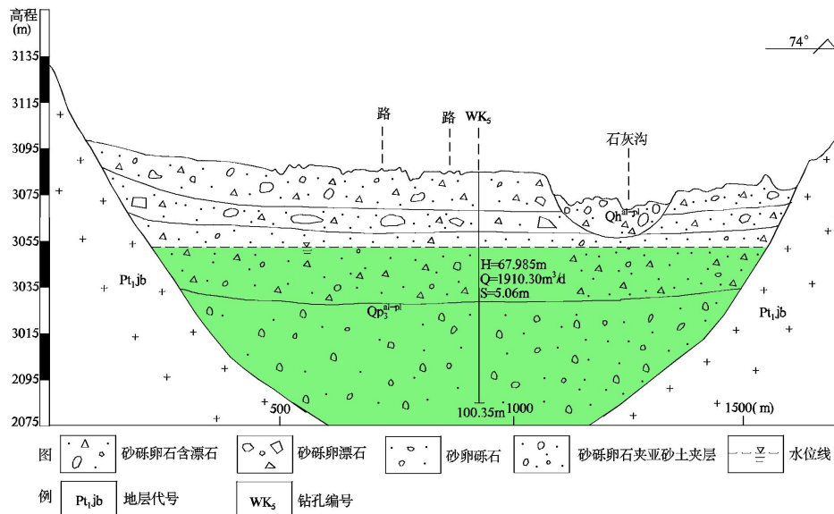
图 9.5.1-3 石灰沟水文地质剖面图
