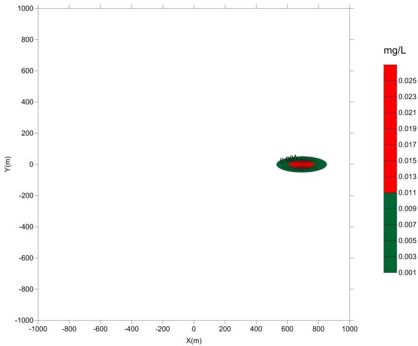
图 9.8.2-2 浓缩池渗漏铅在第四系潜水含水层运移 200d
