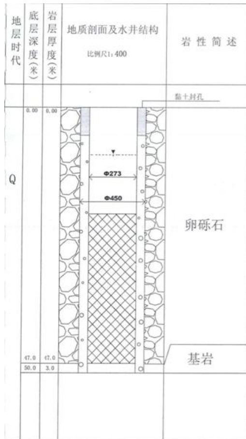
图 9.10.2-5 一选厂下游监测井结构图
